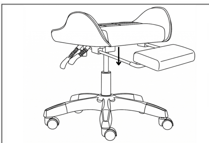
Zamontuj siedzisko z mechanizmem na podstawę
