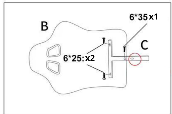
Przymocuj stelaż do oparcia
