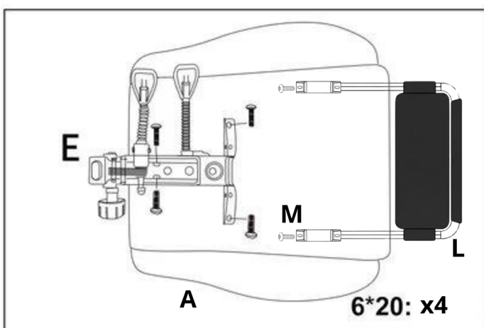
Przymocuj mechanizm od dołu siedziska i zamontuj podnóżek
